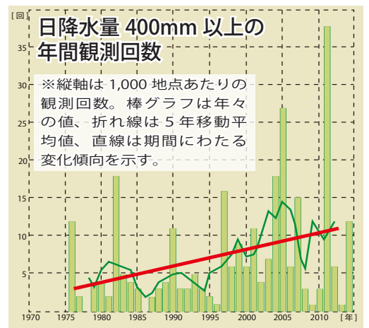
日降水量400 mm 以上の年間観測回数（「気候変動監視レポート2014」全国地球温暖化防止活動推進センターホームページより）
