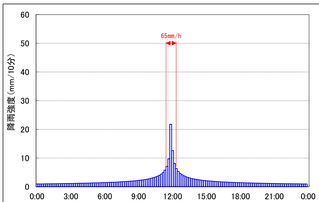
図 5-2 20 年確率降雨（65mm/h）のハイエトグラフ
